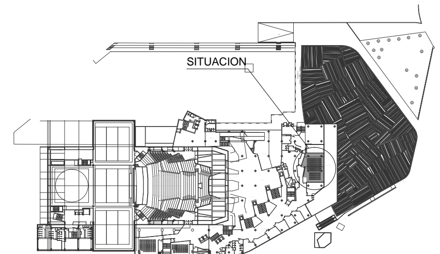
PLANTA 3
